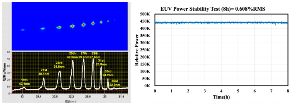
鸞鷲EUV光源实时采集光谱及光谱分析输出, EUV相对功率随时间变化图 (8 小时)
