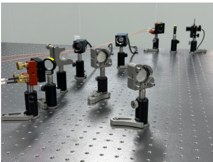
图2 光束指向稳定系统外观图
